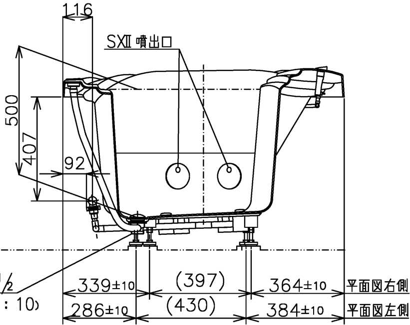
断面A-A
